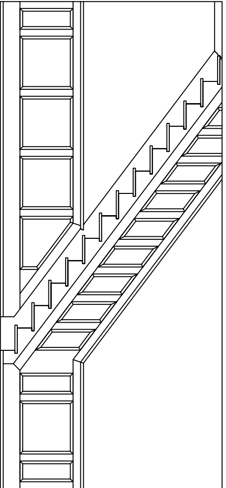
ELEVATION A
