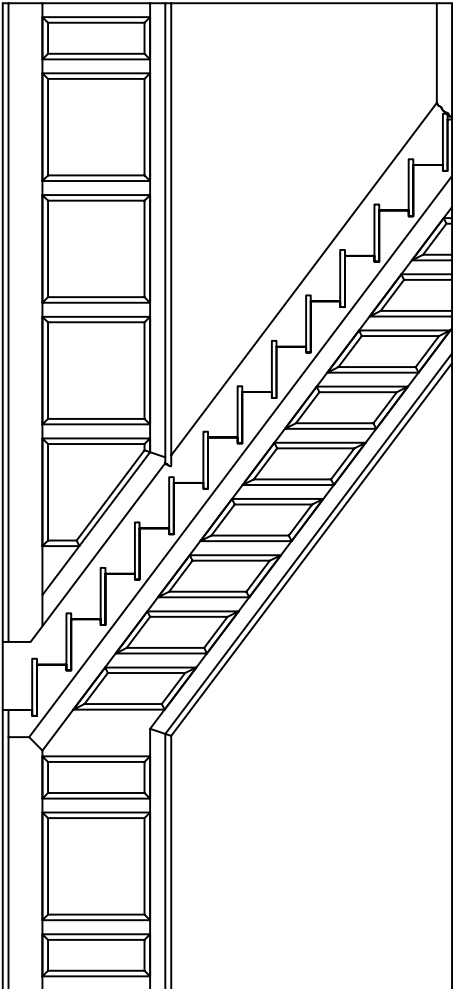
ELEVATION A
